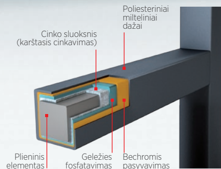
Apsauginio elemento pjūvis „DUPLEX“ sistemoje
