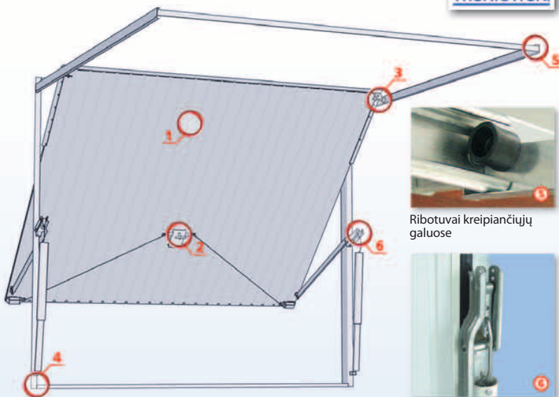
Lengvas spyruoklių įtempimo reguliavimas
