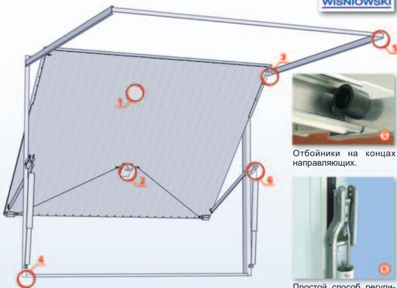
Простой способ регулировки натяжения пружин и самосмазывающиеся подшипники.
